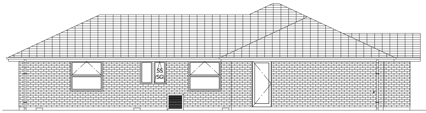
D 4 ELEVATION D 1:100
